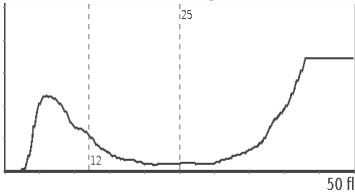
PLT histogram
